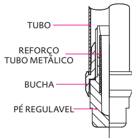
CONJUNTO MONTADO
